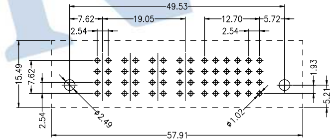
P.C.B Layout
