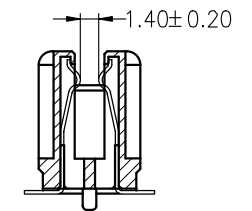
A-A SECTION
